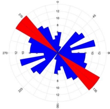
شکل (۶) رزداگرام گسل‌های منطقه‌ی مورد مطالعه
