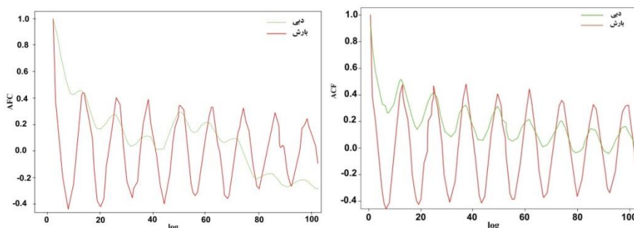
شکل (۱۰) کروئوگرام چشمه روانسر (بالا) و چشمه هولی (پایین)
