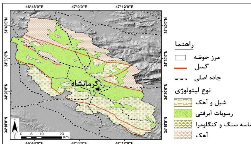
شکل (۳) نقشه طبقاتی پارامترهای زمین‌شناسی
