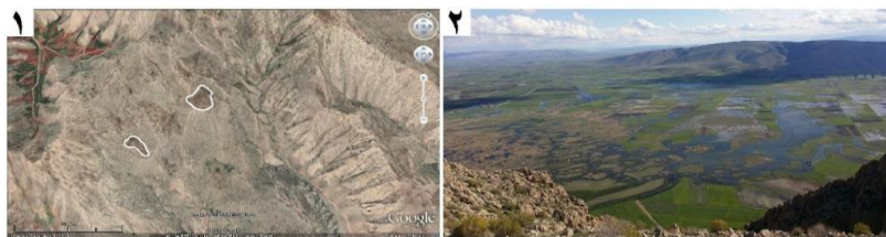
شکل (۹) (۱) تصویر گوگل ارثی از منطقه، (۲) تصویر میدانی منطقه
