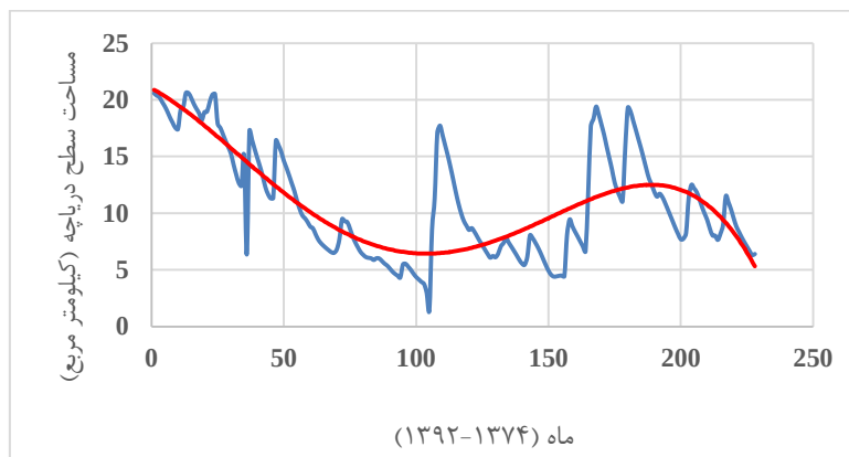
شکل (۵) تغییرات سطح دریاچه برحسب کیلومتر مربع (۱۳۹۴-۱۳۹۲)
