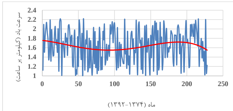
شکل (۴) تغییرات سرعت باد برحسب کیلومتر بر ساعت (۱۳۹۴-۱۳۹۲)
