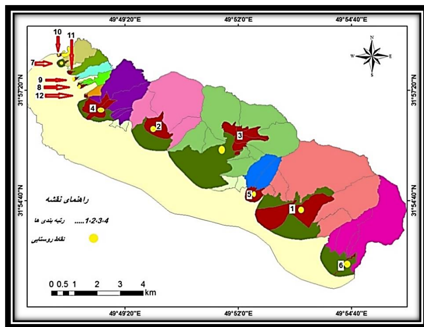
شکل (۴) رتبه بندی خطر وقوع سیلاب در مخروط افکنه های شمال ایذه
