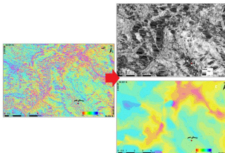
شکل (۴) انجام فیلتر توافقی گلدشتاین بر روی زوج تصویر A_1 از سنجنده ASAR (الف- تداخل نگار فازی مسطح شده ب- تصویر همدوس ج- تصویر تداخل سنجی تفاضلی راداری فیلتر شده)
