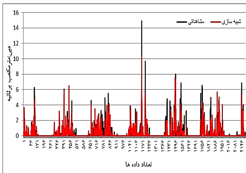
شکل (۶) مقایسه‌ی مقادیر دبی مشاهداتی و شبیه‌سازی‌شده برای دوره‌ی واسنجی در حوضه‌ی آبخیز گرین
