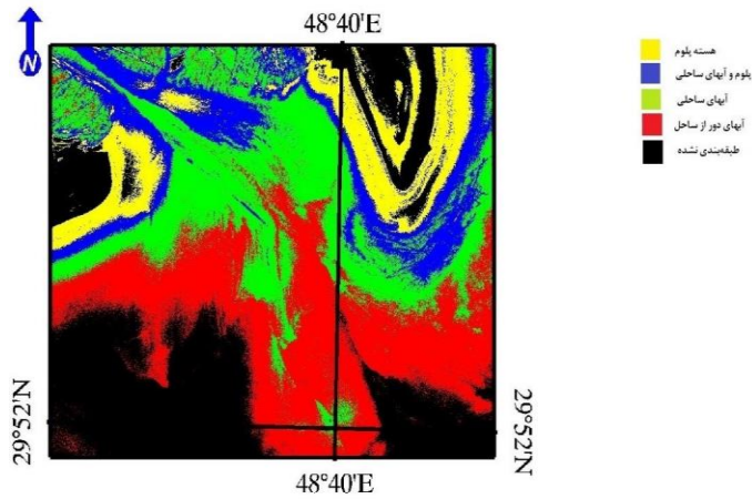
شکل (۱۴) طبقه‌بندی پلوم براساس غلظت مواد معلق (شاخص NSMI) براساس تصویر
