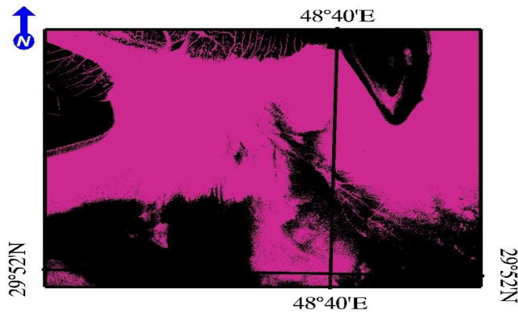
شکل (۱۳) پلوم رودخانه‌ی اروند (با تصویر سنتینل - ۲)
