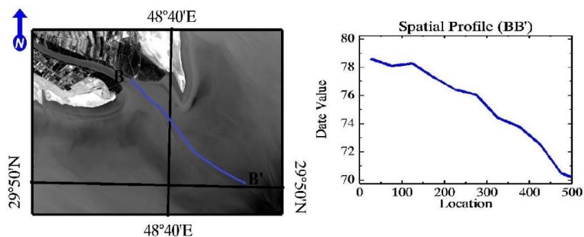
شکل (۴) نیمرخ BB' (رادیانس باند ۲)
