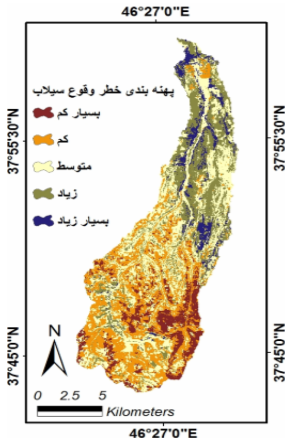
شکل (۱۰) شناسایی حساسیت منطقه نسبت به رخداد سیل
