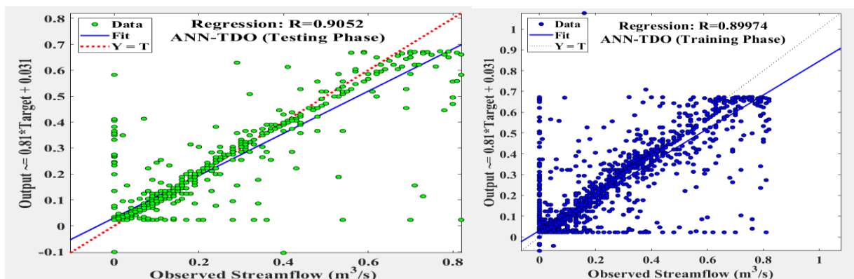
شکل (۳): نمودار پراکنندگی مدل هیبریدی ANN-TDO در دو فاز آموزش و آزمون
