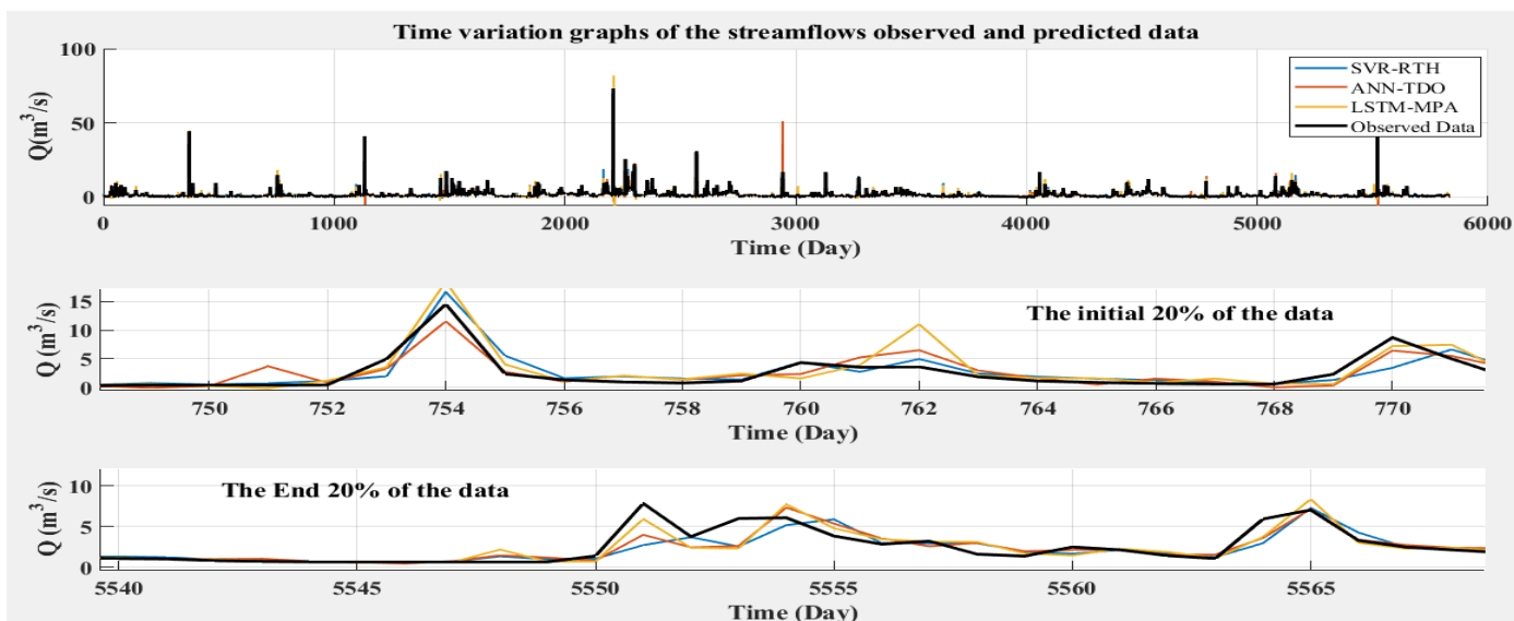
شکل (۶): نمودار سری زمانی داده‌های مشاهده‌ای و پیش‌بینی شده با مدل‌های هیبریدی Figure (6): Time series plot of observed and predicted data for the hybrid models.
