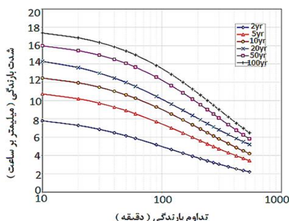
شکل (۴): نمودار توزیع پیرسون تیپ ۳ جهت برآورد بارش طرح
