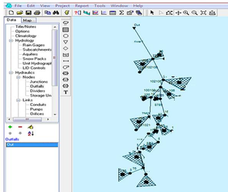
شکل (۶): موقعیت زیرحوضه ها، کانال ها و گره های ارتباطی در زیر حوضه خاکو همدان
