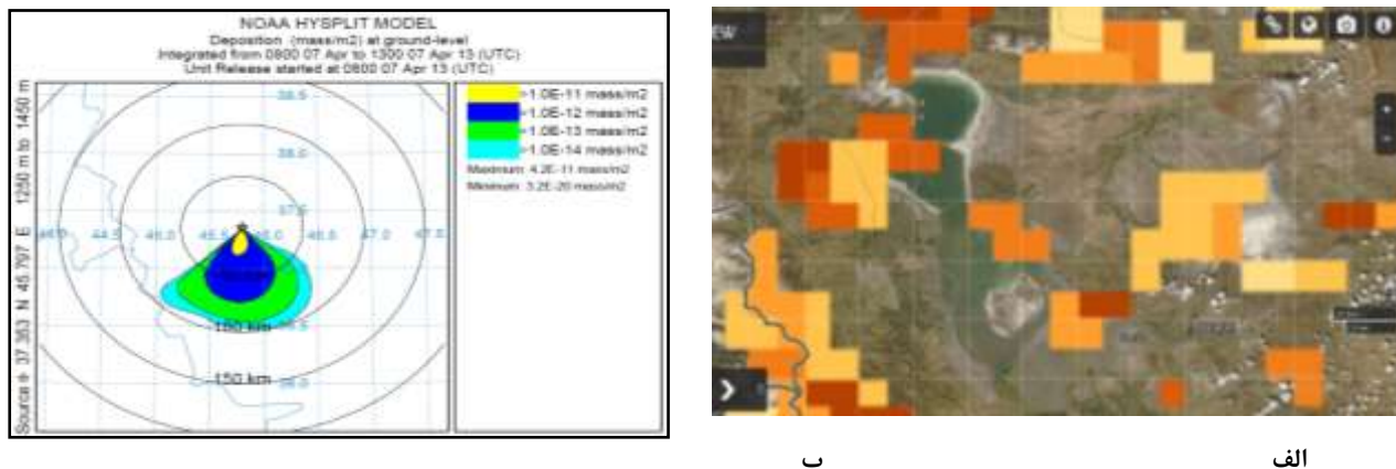
شکل (۱۰): الف) آشکارسازی وقوع توفان ریزگرد در جنوب شرق دریاچه ارومیه با استفاده از شاخص AOD در روز ۰۷ آوریل ۲۰۱۳ (ب): نتیجه اجرای مدل HYSPLIT در شبیه‌سازی مسیر و مسافت انتشار ریزگردها در روز ۰۷ آوریل ۲۰۱۳
