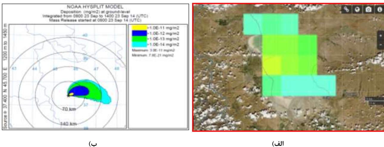
شکل (۱۱): الف) آشکارسازی وقوع توفان ریزگرد در جنوب شرق دریاچه ارومیه با استفاده از شاخص AOD در روز ۲۳ سپتامبر ۲۰۱۴ (ب): نتیجه اجرای مدل HYSPLIT در شبیه‌سازی مسیر و مسافت انتشار ریزگردها در روز ۲۳ سپتامبر ۲۰۱۴
