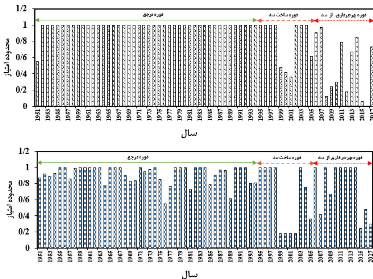
شکل (۵): تغییرات زمانی انحراف شاخص‌های جریان‌های حداکثر (High Monthly flow (HM) (بالا)، و حداقل ماهانه (Lowest monthly flow (LM) (پایین)، رودخانه شهرچای در دوره‌های مختلف Figure (5): Temporal variations of the Highest Monthly flow (HF) (top), and Lowest Monthly flow (LM) (down), in Shahrchai River across different periods
