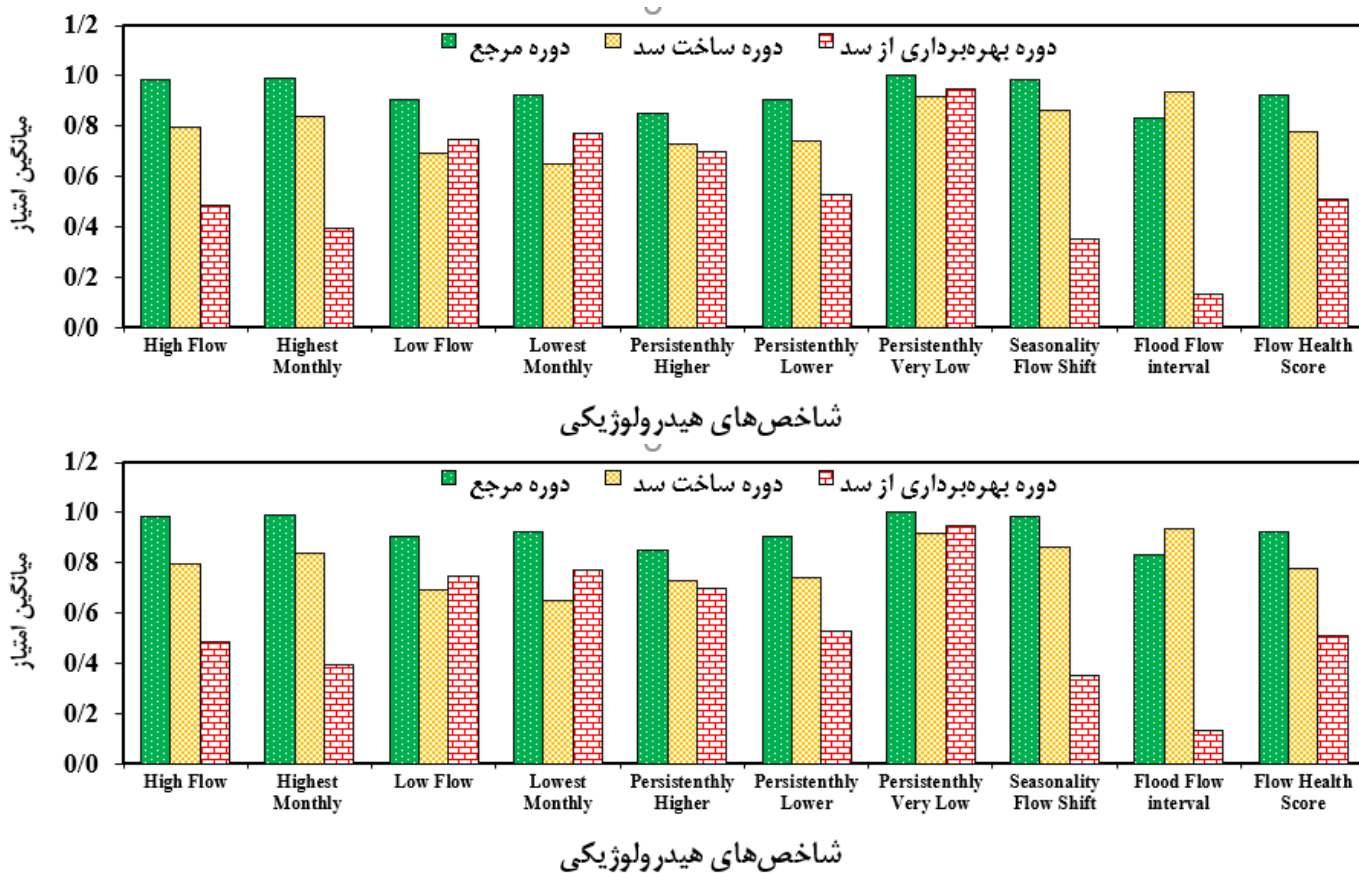
شکل (۹): میانگین تغییرات زیرشاخص‌ها و شاخص‌های سلامت هیدرولوژیک جریان در رودخانه شهرچای در دوره‌های زمانی مختلف Figure (9): Changes in the average values of sub- indicators and flow health scores in Shahrchay River in different time periods
