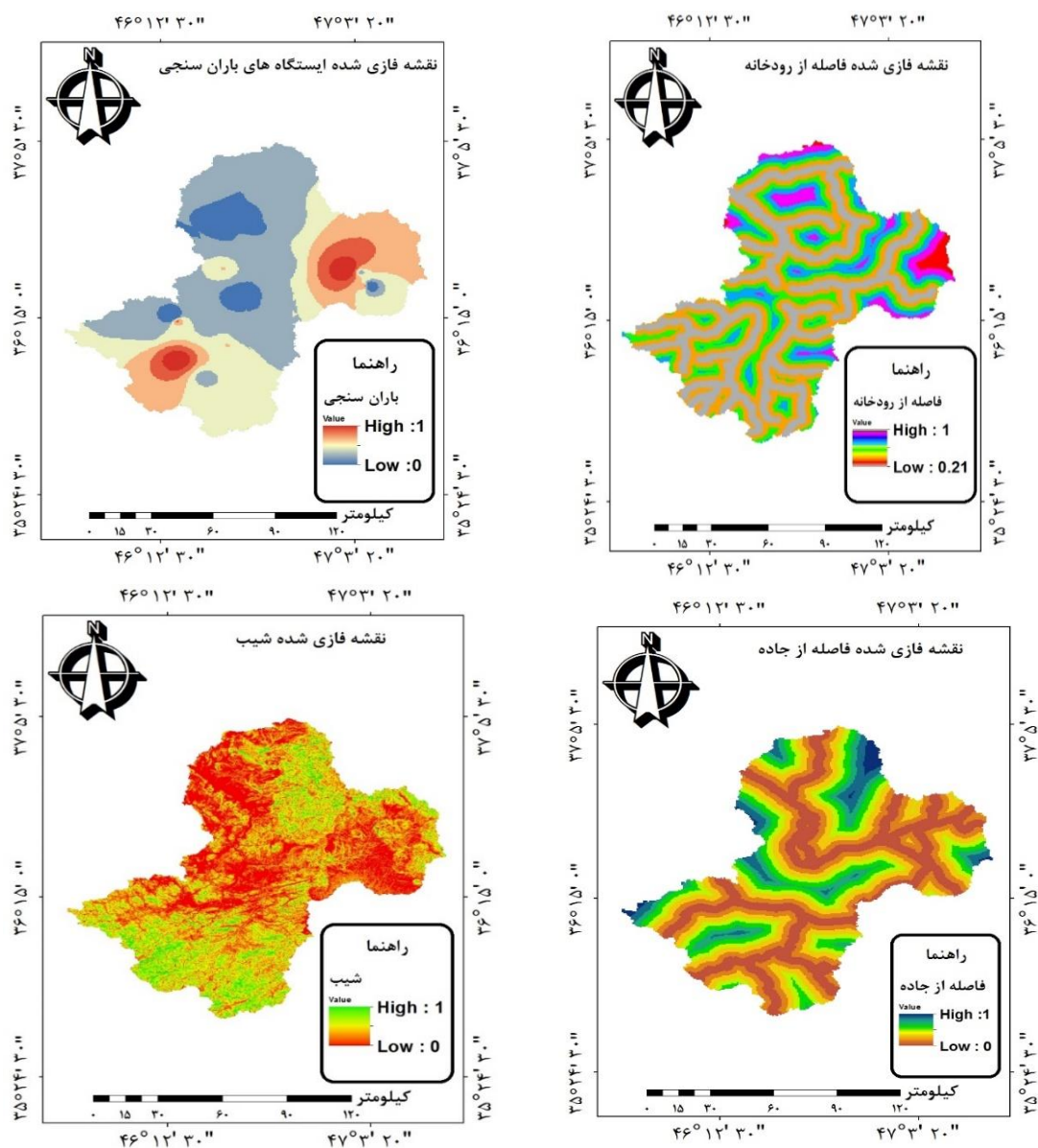
شکل (۱۰): متغیرهای مورد استفاده جهت تولید نقشه‌ی فرسایش خاک
