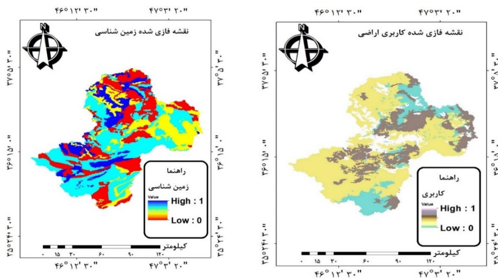
ادامه‌ی شکل (۱۰): متغیرهای مورد استفاده جهت تولید نقشه‌ی فرسایش خاک
