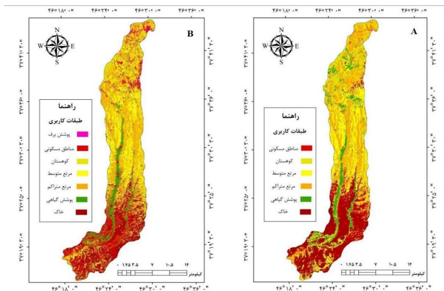
شکل (۴) نقشه‌ی طبقه‌بندی کاربری اراضی به روش پیکسل پایه (A و B: روش حداقل فاصله به ترتیب برای سال ۲۰۰۰ و ۲۰۲۰. Figure (4): Land use classification map by basic pixel method (A and B: minimum distance method for 2000 and 2020,
