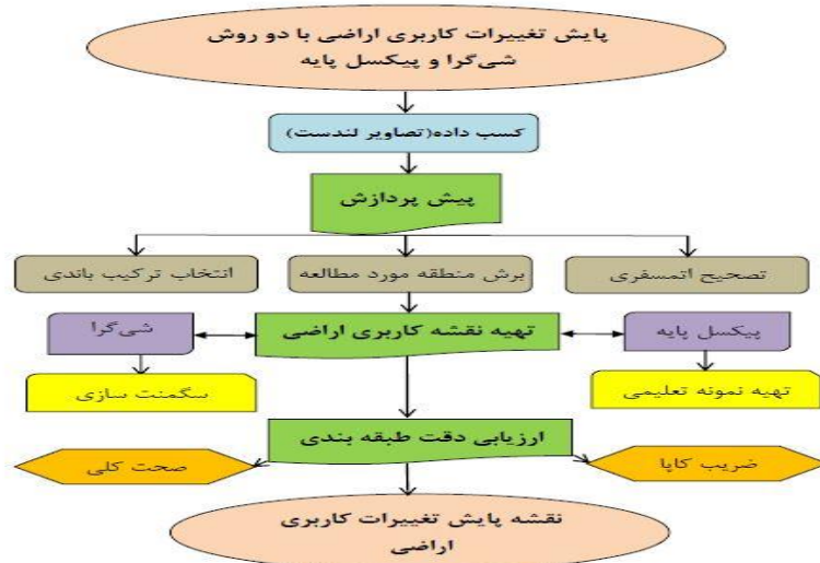
شکل (۲): مراحل و روند پژوهش Figure (2): Steps and process of research
