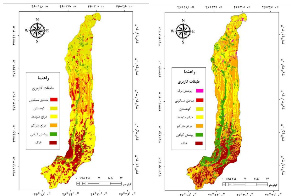
شکل (۵): نقشه‌ی طبقه‌بندی کاربری اراضی به روش شی‌گرا برای سال‌های ۲۰۰۰ (سمت چپ) و ۲۰۲۰ (سمت راست)
