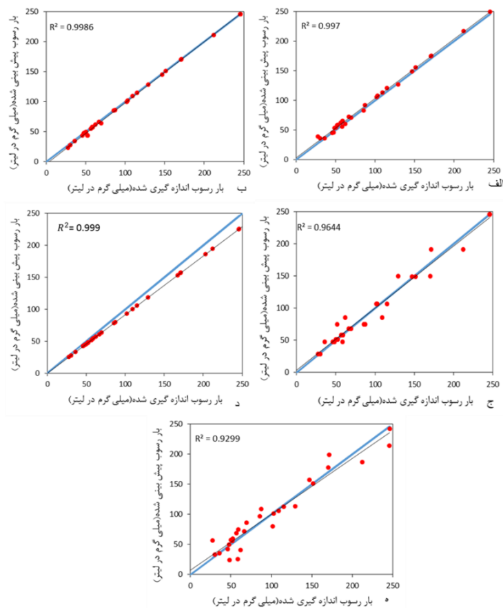
شکل (۶): نمودار پراکنندگی مقادیر مشاهده شده و پیش‌بینی شده‌ی بار رسوب معلق توسط مدل‌های الف: شبکه عصبی مصنوعی، ب: ماشین بردار پشتیبان تکاملی، ج: درخت تصمیم M5، د: فرآیند گوسی، ه: رگرسیون، با در نظر گرفتن پارامترهای فیزیوگرافی
