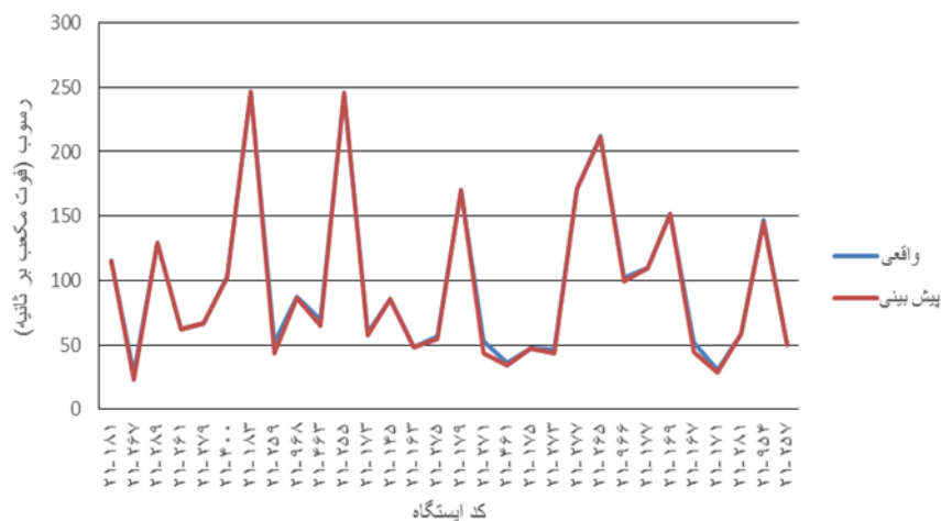
شکل (۷): مقادیر واقعی و پیش‌بینی شده توسط مدل ماشین بردار پشتیبان تکاملی با در نظر گرفتن پارامترهای فیزیوگرافی Fig (7): Actual and Predicted Values by the Evolutionary Support Vector Machine Model Considering the physiographic parameters
