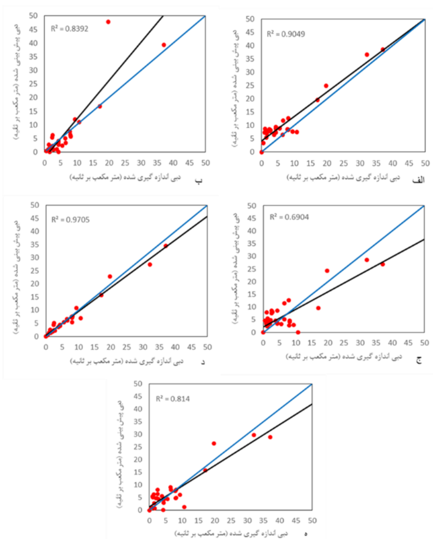
شکل (۲): نمودار پراکندگی مقادیر مشاهده شده و پیش‌بینی شده دبی توسط مدل‌های الف: شبکه عصبی مصنوعی، ب: ماشین بردار پشتیبان تکاملی، ج: درخت تصمیم M5، د: فرآیند گوسی، ه: رگرسیون
