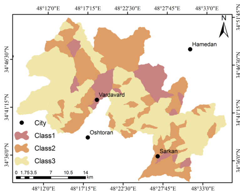
شکل (۴) وضعیت شاخص عدم تقارن در زیرحوضه‌های الوند همدان Fig (4) Status of asymmetry index in Alvand sub-basins of Hamedan
