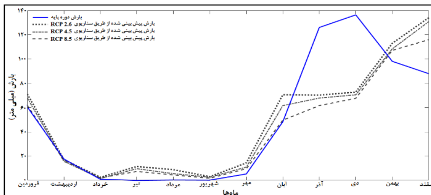
شکل (۷) نمودار مقادیر بارش ماهانه شبیه‌سازی شده برای سال ۲۰۰۶-۲۱۰۰ با به کارگیری سناریوهای RCP 2.6 - RCP 4.5 و RCP 8.5
