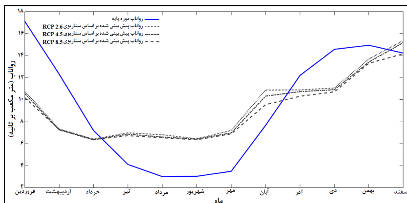
شکل (۱۱) نمودار مقادیر رواناب ماهانه شبیه‌سازی شده برای سال ۲۰۰۶-۲۱۰۰ با به کارگیری سناریوهای RCP 2.6 و RCP 4.5 و RCP 8.5
