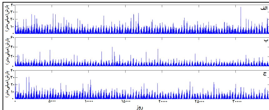
شکل (۶) نمودار مقادیر بارش روزانه شبیه‌سازی شده برای سال ۲۰۰۶-۲۱۰۰ با به کارگیری سناریوهای RCP 2.6 - الف: RCP 2.6 - ب: RCP 4.5 و ج: RCP 8.5
