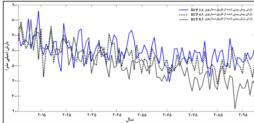
شکل (۸) نمودار مقادیر بارش سالانه شبیه‌سازی شده برای سال ۲۰۰۶-۲۱۰۰ با به کارگیری سناریوهای
