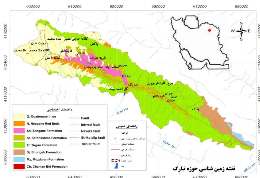
شکل (۱) نقشه‌ی زمین‌شناسی و موقعیت جغرافیایی حوضه‌ی آبریز تبارک‌آباد (اقتباس از نقشه با مقیاس ۱:۱۰۰۰۰۰؛ فوچان سازمان زمین‌شناسی کشور، قائمی، ۱۳۸۳) و تعیین شماتیک بعضی از پارامترهای مورفومتری بر روی آن
