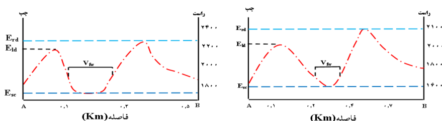
شکل (۴) نمایش وضعیت شاخص (V_f) نسبت به پهنای کف دره به ارتفاع دره (V_{fw}) در دو مقطع از حوضه‌ی آبریز تبارک‌آباد الف: مقطعی از زیرحوضه‌ی یدک و ب: مقطعی از زیرحوضه‌ی زیرآبه
