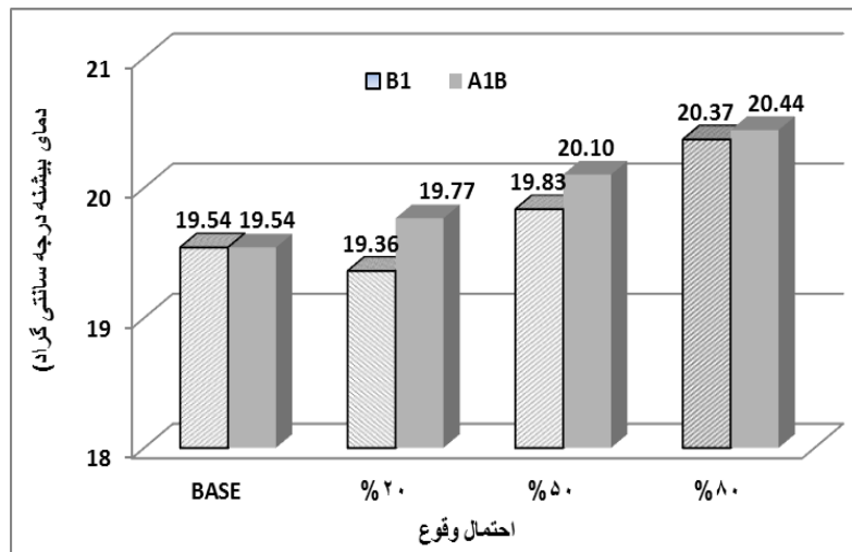
شکل (۱۱) تغییرات سالانه بیشینه‌ی دما در احتمال وقوع مختلف سناریوی B1 و A1B
